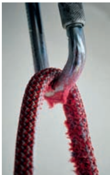
Scheuermann: Nur nach dem Zufügen von Chalk konnten wir den Seilen etwas »anhaben«.
