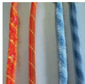
Aufreibend: die gleichen Seile mit dem Einsatz von Chalk (links) und ohne nach jeweils 150 Scheuerzyklen
